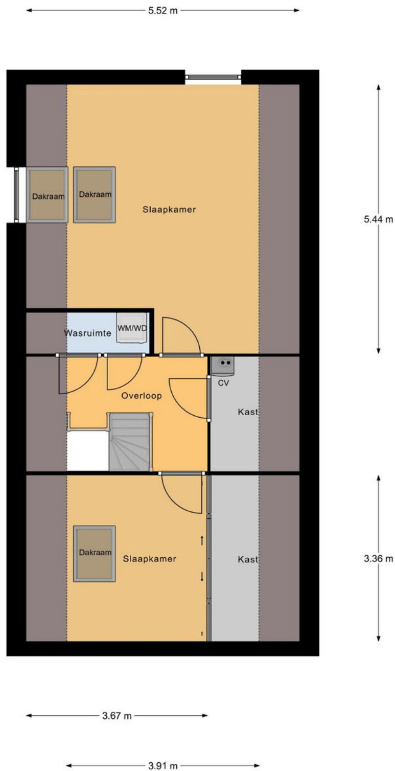
2e Verdieping
